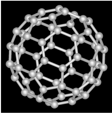
chimie (fullerène C60)
